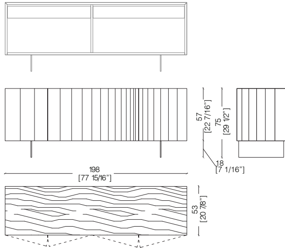
ST 12 LG low sideboard - credenza bassa - niedrige anrichte - buffet bas - Низкая кренца
