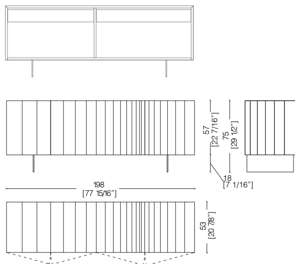
ST 12 MG low sideboard - credenza bassa - niedrige anrichte - buffet bas - Низкая кренца
