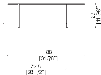
BD 323 coffee table - tavolino niedriger tisch - table basse - Журнальный столик
