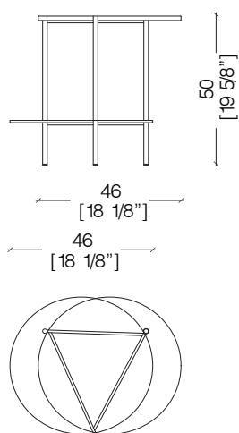
BD 333 coffee table - tavolino niedriger tisch - table basse - Журнальный столик
