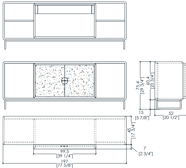
TAL D23 low storage unit - mobile contenitore basso - niedriges behältermöbel - meuble conteneur bas - Низкий шкаф
