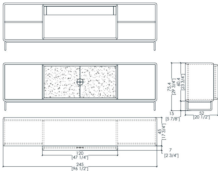
TAL D24 low storage unit - mobile contenitore basso - niedriges behältermöbel - meuble conteneur bas - Низкий шкаф
