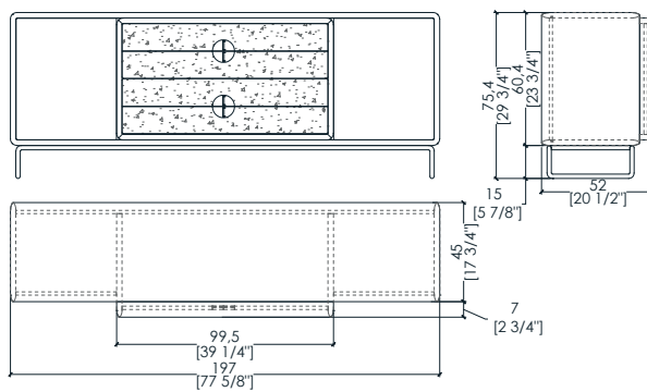
TAL C33 low storage unit - mobile contenitore basso - niedriges behältermöbel - meuble conteneur bas - Низкий шкаф
