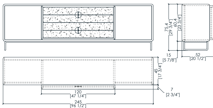
TAL C34 low storage unit - mobile contenitore basso - niedriges behältermöbel - meuble conteneur bas - Низкий шкаф
